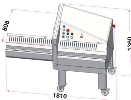
Dimensions ICÔNE 700
